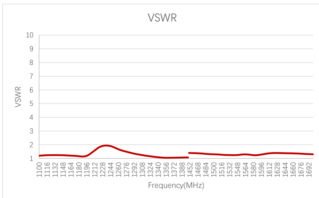
VSWR
